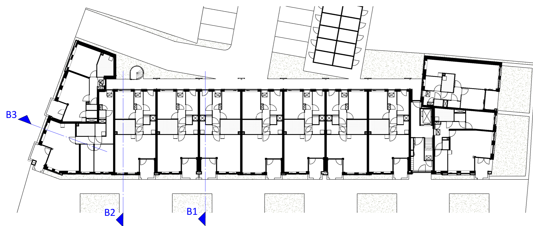
BEGANE GROND 1 : 300
