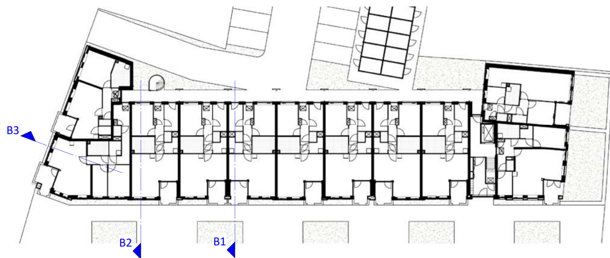
BEGANE GROND 1 : 300
