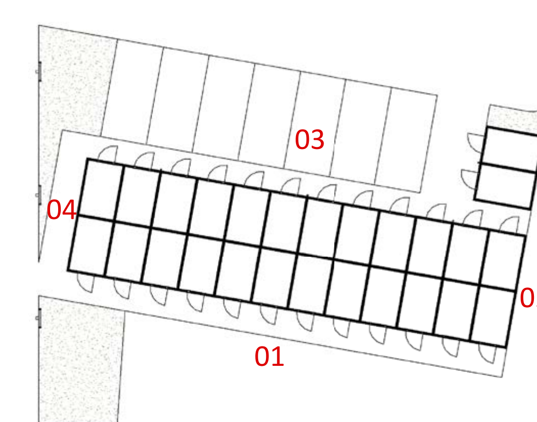
BEGANE GROND 1 : 200
